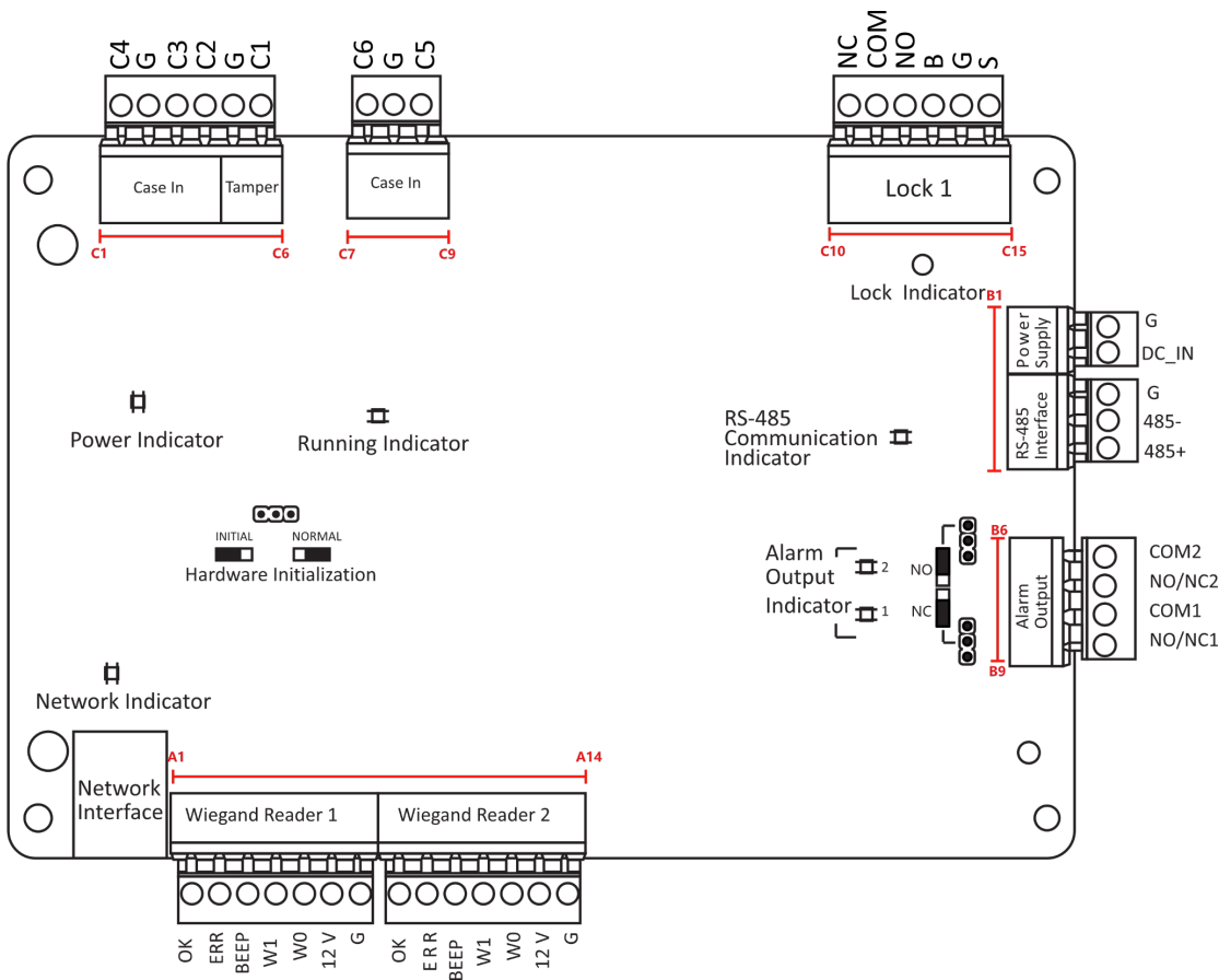
Рисунок 4-1. Основная плата управления контроллера доступа на 1 дверь
