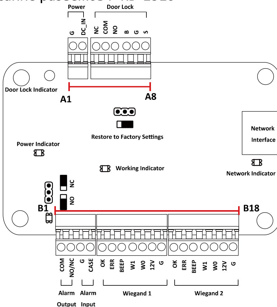
Описание разъемов F-KD-1310
